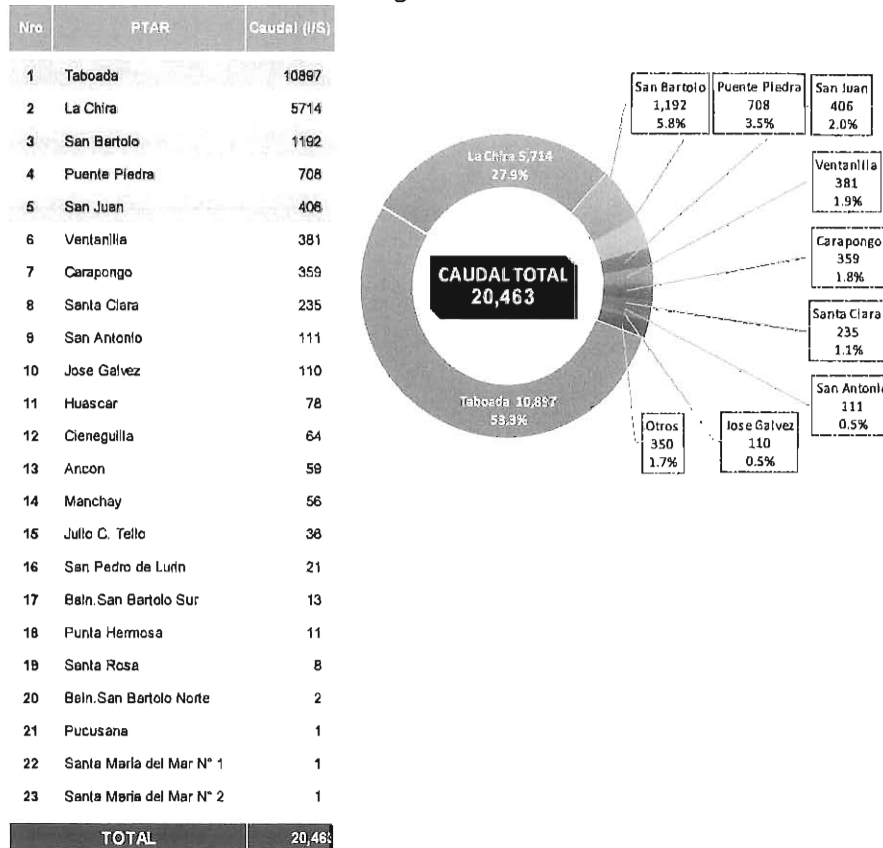
Cuadro N° 9 Caudal de Tratamiento de Aguas Residuales (l/s) Al Segundo Trimestre 2020
